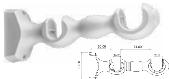
DUPLO MÉDIO/ GROSSO PARA ILHÓS 61CP 19mm/28mm
