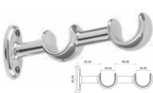
DUPLO GROSSO S028 28mm/28mm
