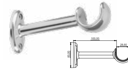
GROSSO ALONGADO SGA10 28mm
