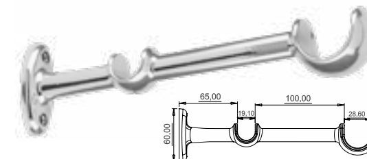
DUPLO ALONGADO MÉDIO/GROSSO SGE06 19mm/28mm
