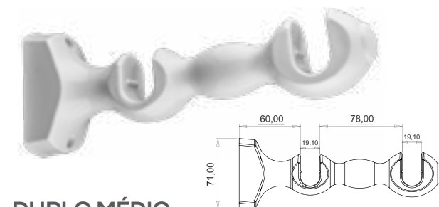
DUPLO MÉDIO PARA ILHÓS 41CP 19mm/19mm
