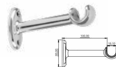
MÉDIO ALONGADO SMA10 19mm
