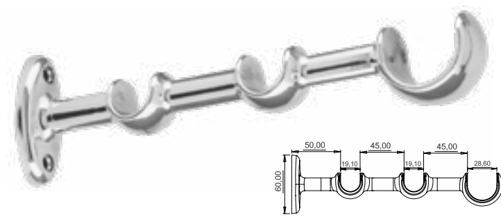
TRIPLO MÉDIO/MÉDIO/GROSSO S08 19mm/19mm/28mm
