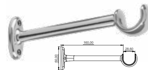
MÉDIO ALONGADO SGA15 19mm
